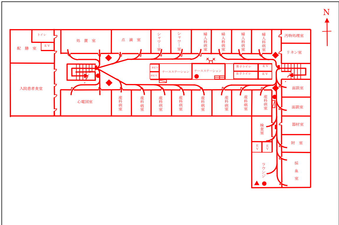
1 1階平面図
